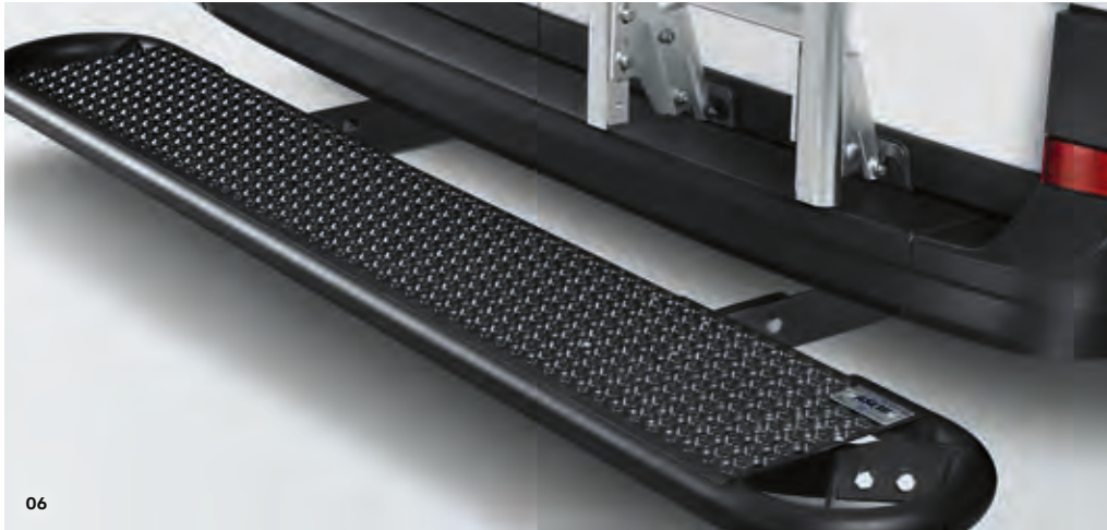
06 Marchepied suspendu, à l’arrière. La suspension par ressorts à lames permet d’amortir les petits chocs. | VA | PC | PL | CH |
